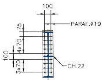
SEÇÃO (A)
