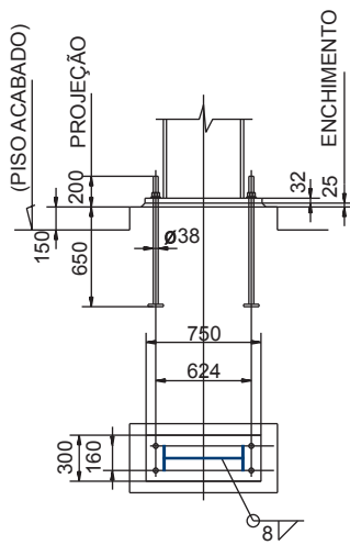
BASES TIPOS I & II
