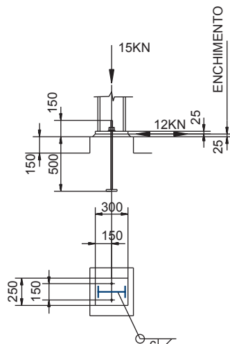
BASES TIPO III (COLUNAS DE FECHAMENTO)
