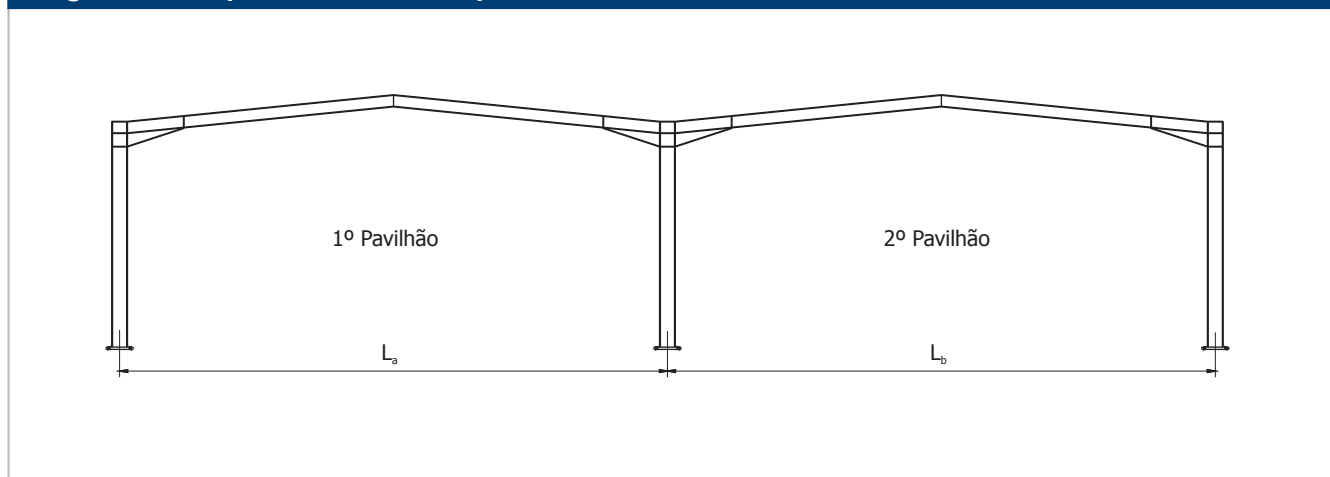
Figura 3 - Galpão de Vãos Múltiplos
