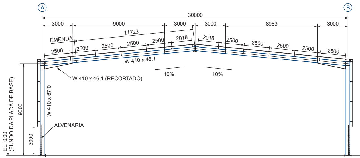
SEÇÃO TRANSVERSAL
