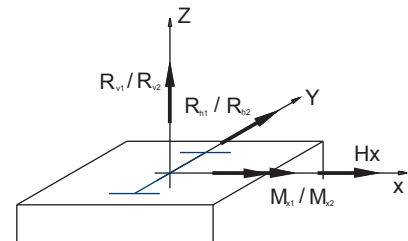
DIREÇÃO POSITIVA DOS ESFORÇOS
