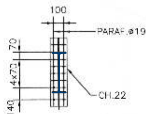
SEÇÃO (B)
