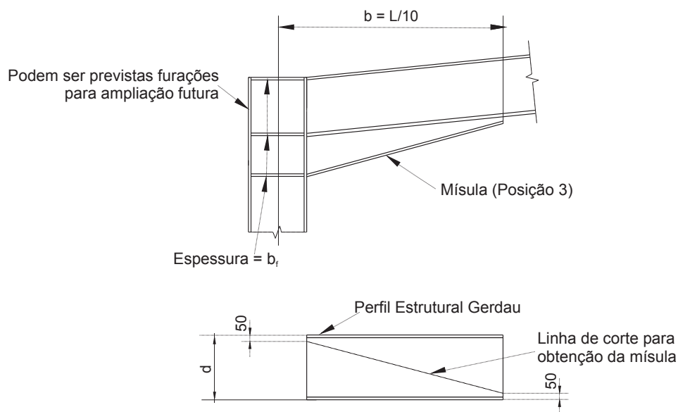
Figura 8 - Nó do Pórtico e Recorte das Mísulas
