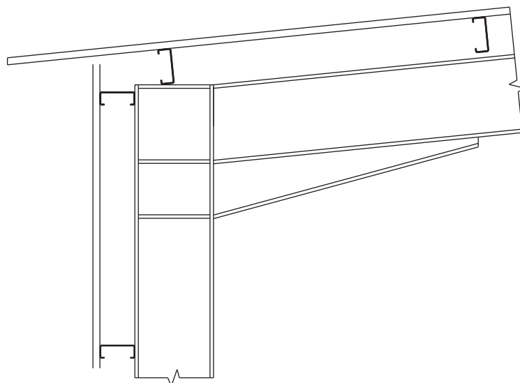
Figura 15 - Detalhe para Galpão com Fechamento sem Calha
