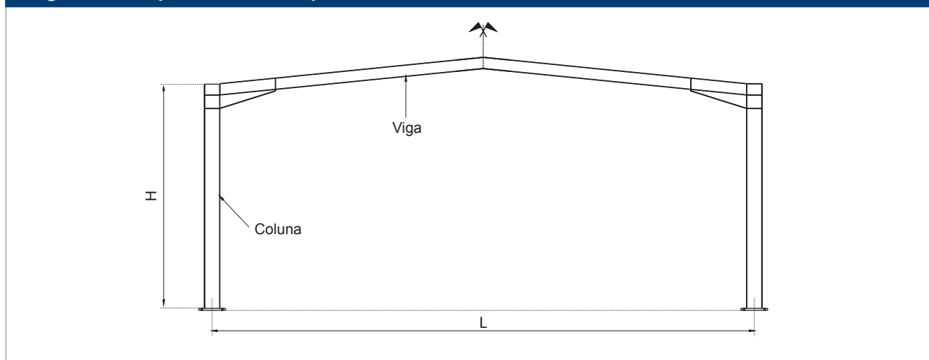
Figura 2 - Galpão de Vão Simples
