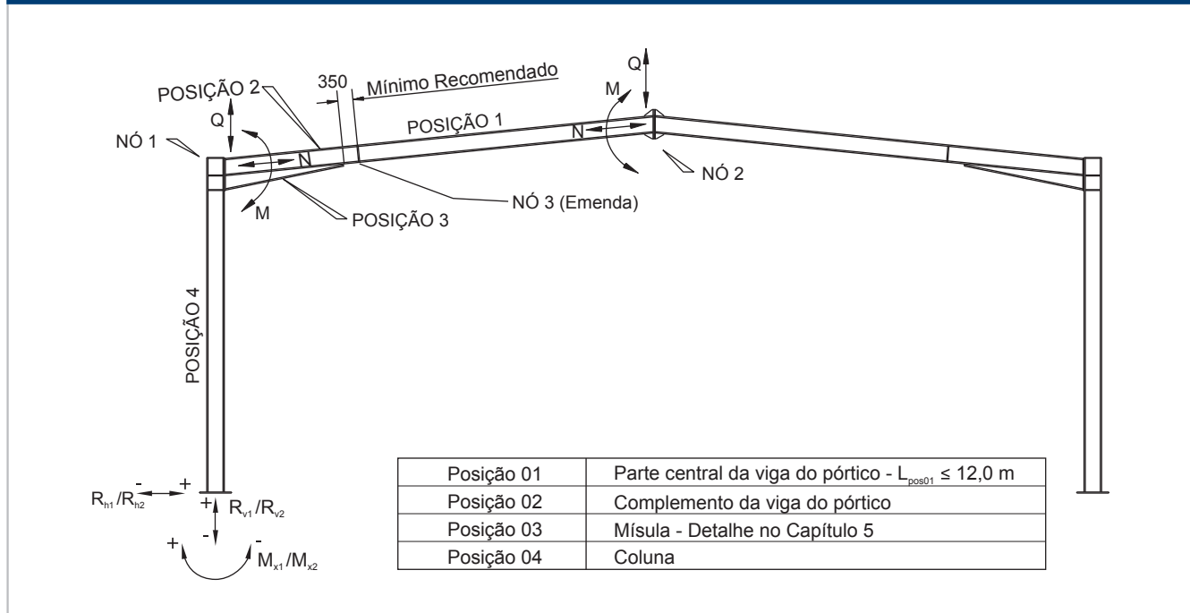
Figura 16 - Composição Geométrica
