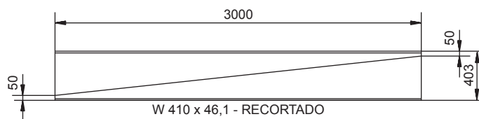
DET. PARA RECORTE DAS MÍSLAS
